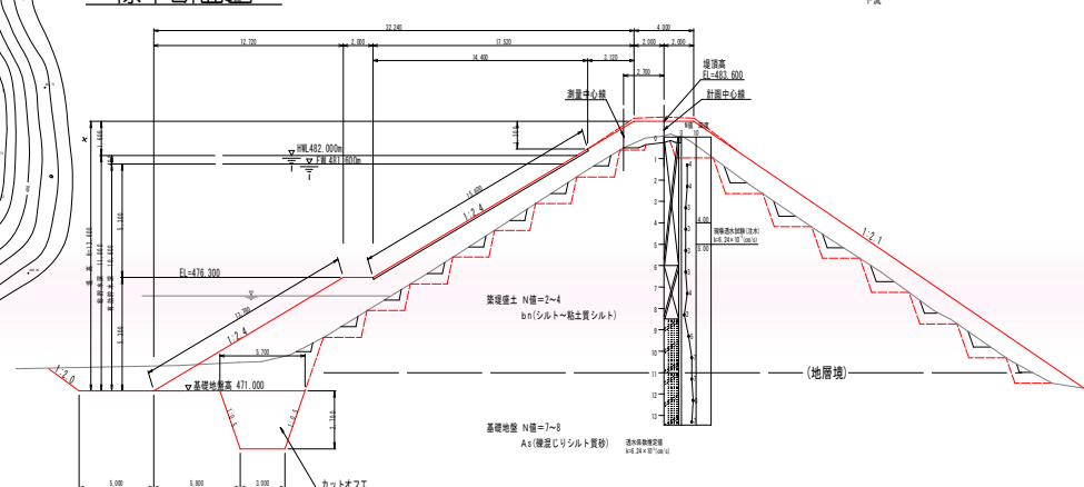
標準断面図
